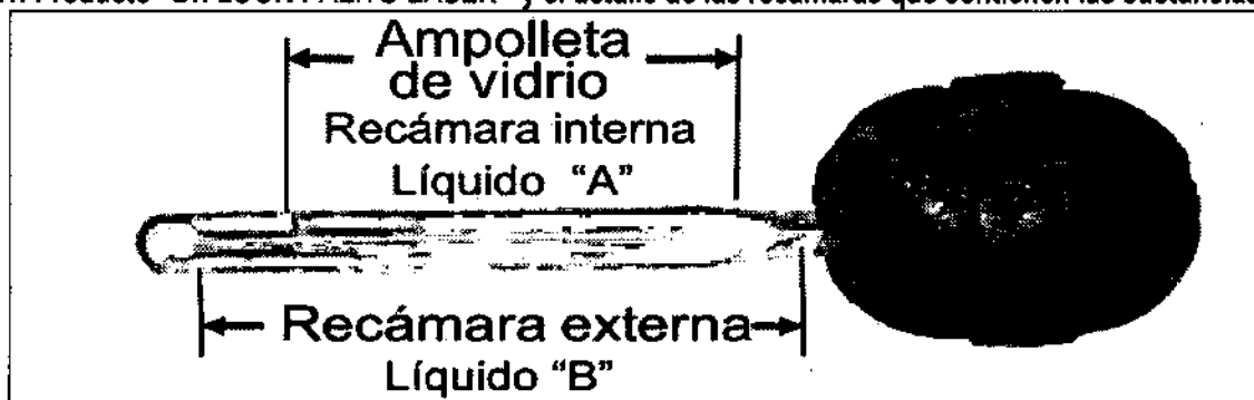
Imagen 21. Producto "Dr. LOOK PALITO LÁSER" y el detalle de las recámaras que contienen las sustancias químicas
