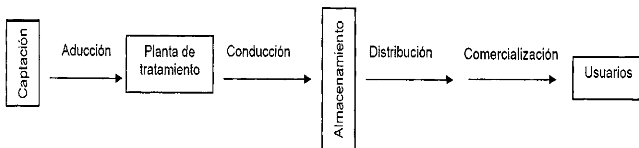
Figura No. 2 Mapa del proceso productivo del sistema de acueducto
